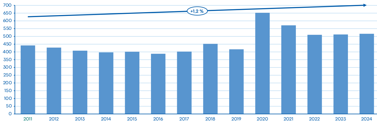
Počet předpisů publikovaných ve Sbírce zákonů (ČR, po letech)
