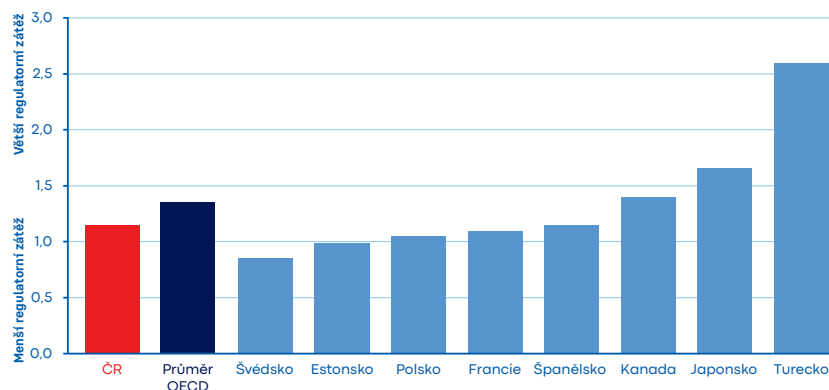
Index celkové regulační zátěže ekonomiky (OECD, 2023, PMR indicator)
