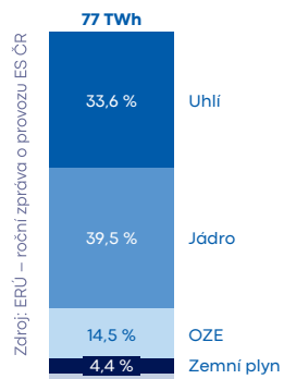
Výroba elektřiny v ČR brutto (2023)
